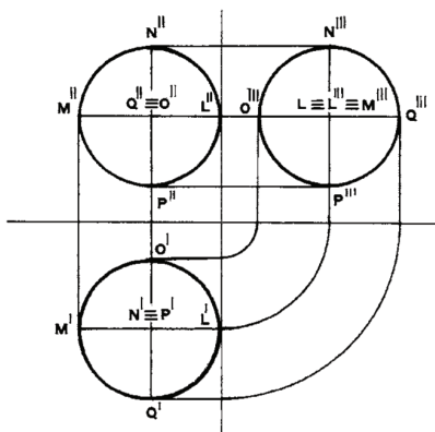
3 Proiezione ortogonale di una sfera che poggia sul PL
