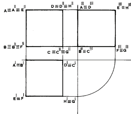
2 Cubo che poggia sul PV con una faccia
