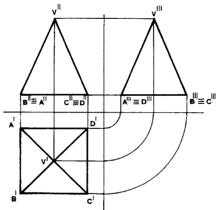
1 Proiezione ortogonale di una piramide a base quadrata sospesa tra i piani di proiezione e con la base parallela al PO
