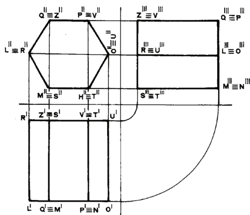
5 Proiezione ortogonale di un prisma a base esagonale sospeso tra i piani e avente la base parallela al PV
