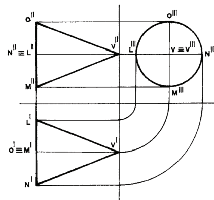
4 Proiezione ortogonale di un cono retto che poggia sul PL con il vertice e avente la base parallela al PL
