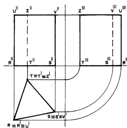
6 Proiezione ortogonale di un prisma a base triangolare poggiato sul PO con la base e posto obliquamente rispetto ai piani PV e PL
